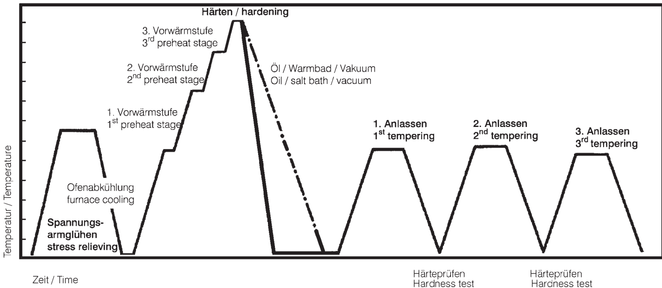
Wärmebehandlungsschema
